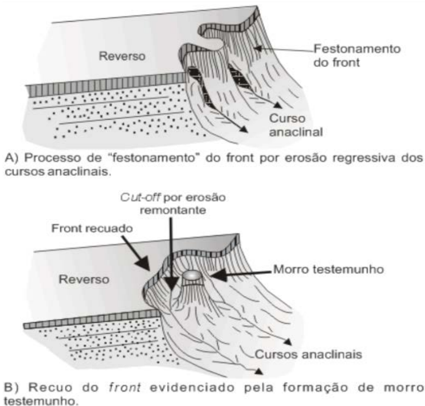
Figura 4 – Esquema de recuo do front em hogbacks , segundo Casseti (2005)
