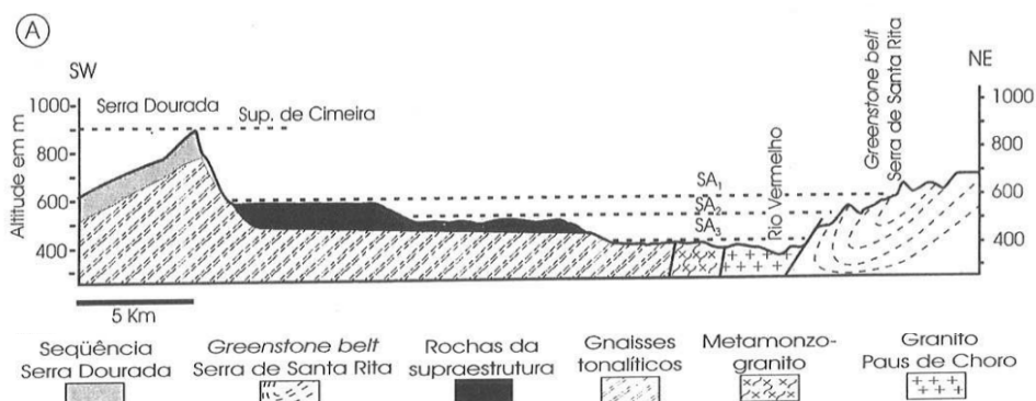
Figura 3 – Arranjo Geolgico da seo Serra Dourada, superfcie intermontana e Serra de Santa Rita, de acordo com Jost et al. (2005)
