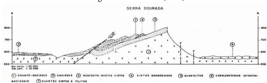
Figura 1 – Arranjo geológico da Serra Dourada segundo Danni et al. (1973)
