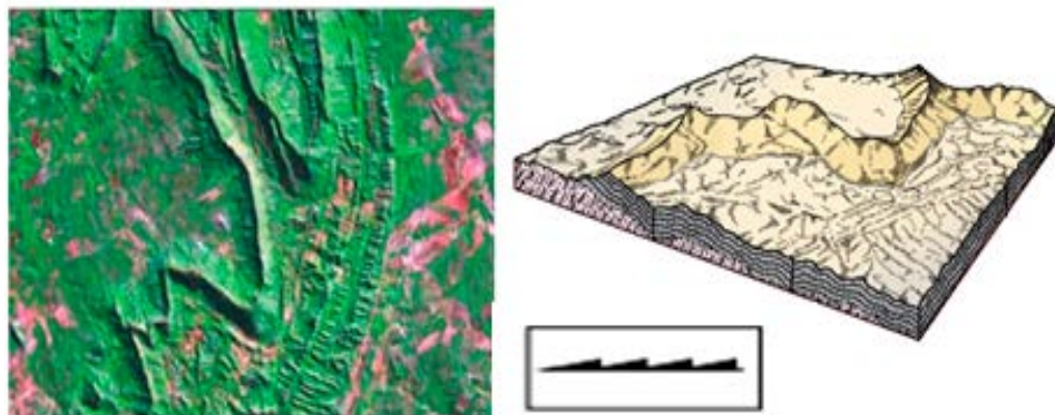
Figura 1 – Relevo tipo hogback
